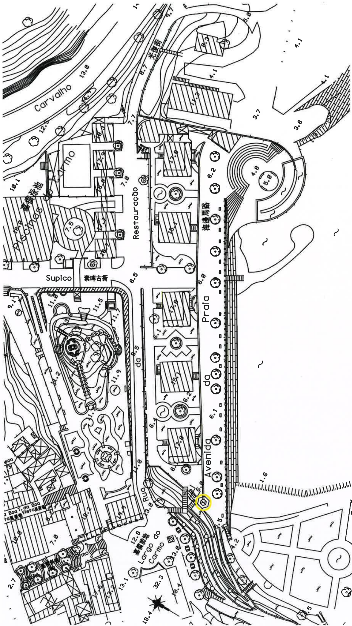
Anexo VII: Planta de localização do quiosque das Casas da Taipa
